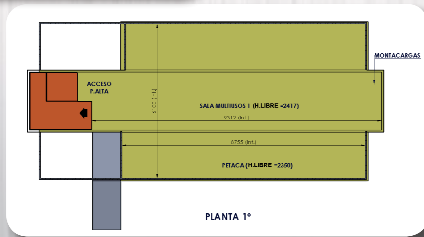
SUPERFICIE ÚTIL PRIMERA PLANTA
